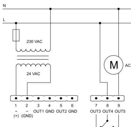
Příklad zapojení čidla TVOC se dvěma relé (2x spínací kontakt)
